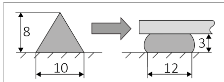
Figura 1: Configurazione consigliata del cordone
