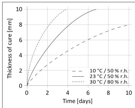
Grafico 1: Velocità di vulcanizzazione di SikaTack® Panel-50
